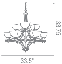
26132 Ambrato Chandelier 9Lt x 40w Halogen 120v JCD (G-9 Base) Finish ABRZ Glass AMB Included 5ft Chain & 10ft Wire CUL Dry
