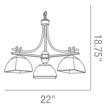
26123 Ambrato Chandelier 3Lt x 40w Halogen 120v JCD (G-9 Base) Finish ABRZ Glass AMB Included 5ft Chain & 10ft Wire CUL Dry
